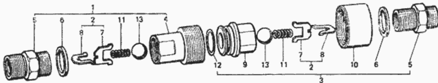
Рис. 138. Устройство запорное 3057-4616320
